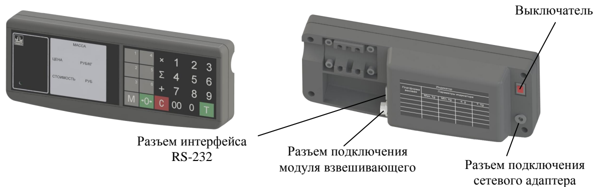
Рис. 2.1 – Терминал Т/ТВ
