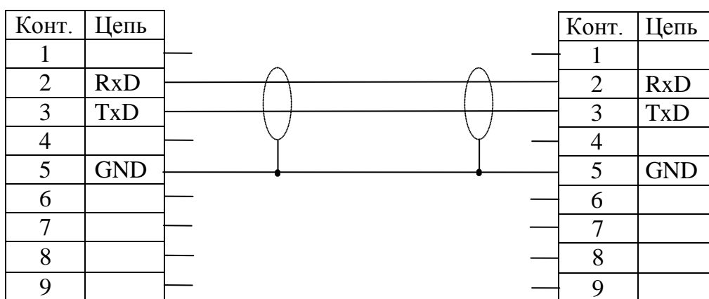
Рис. 6.3 – Схема электрическая кабеля для варианта весов с розеткой DB-9F
