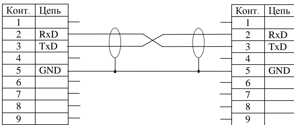
Рис. 6.2 – Схема электрическая кабеля для варианта весов с вилкой DB-9M
