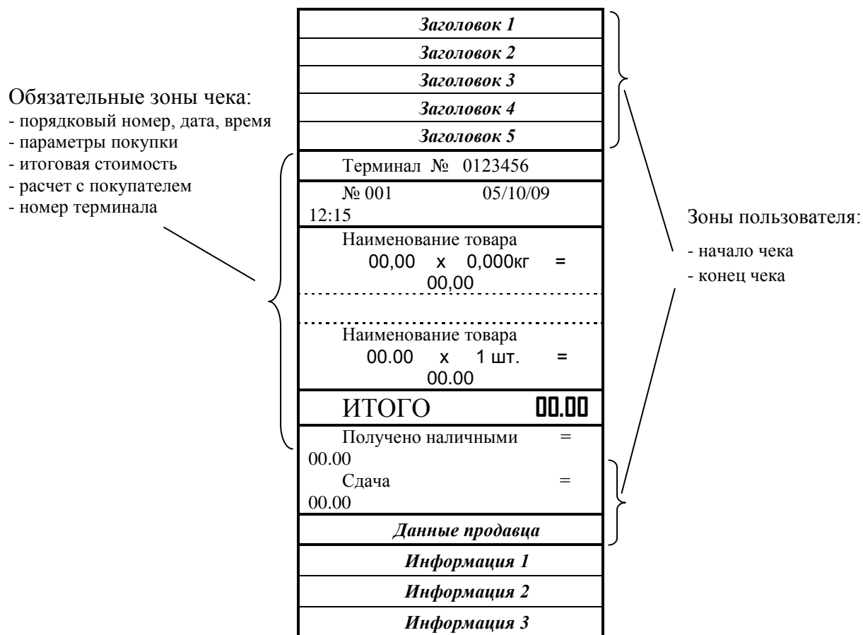
Рис. 8.3 - Структура товарного чека
